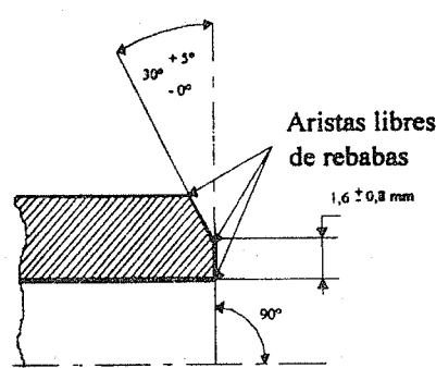
Figura 2 - Extremos biselados
